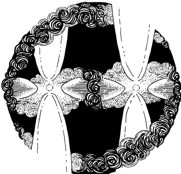
Inclination
